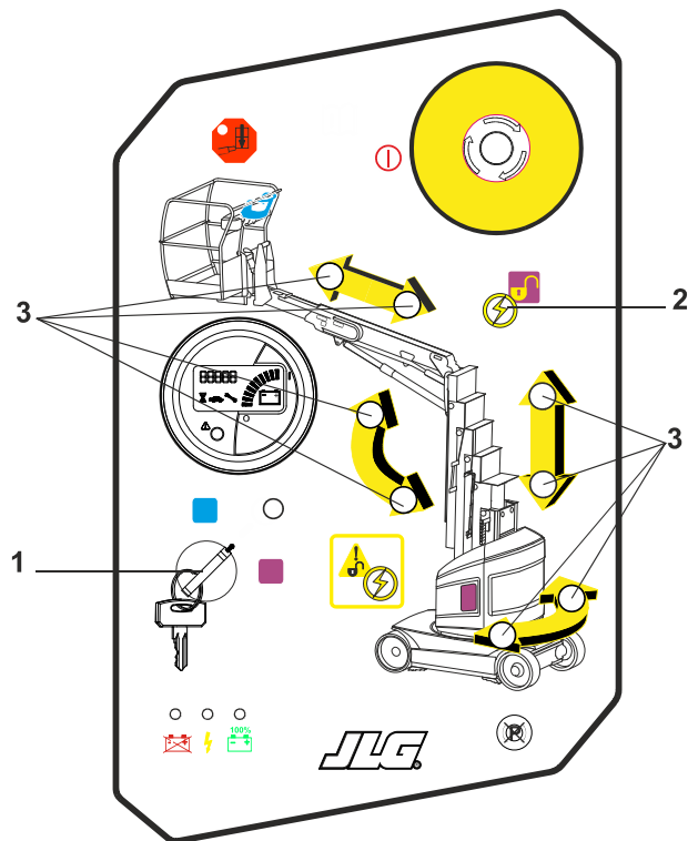
Figura 4-1. Controles de Emergencia
