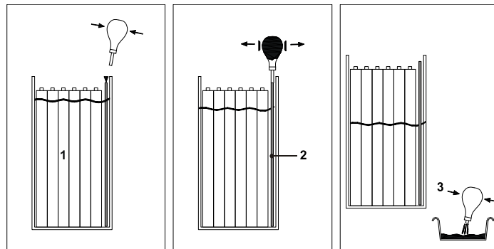
Figura 5-7. Drenar el agua
