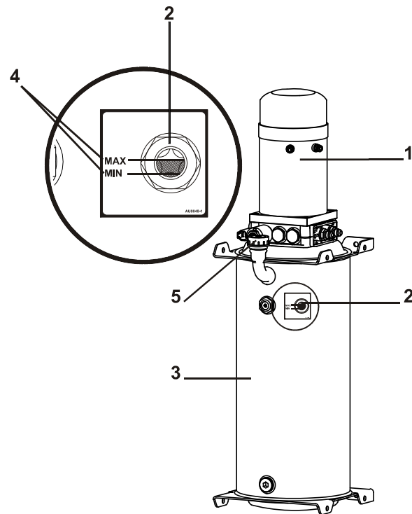
Figura 5-9. Comprobación de la aceite hidráulico
