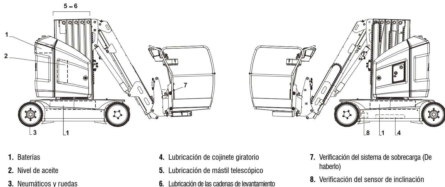
Figura 5-3. Mantenimiento del Operador y Diagrama de Lubricación
