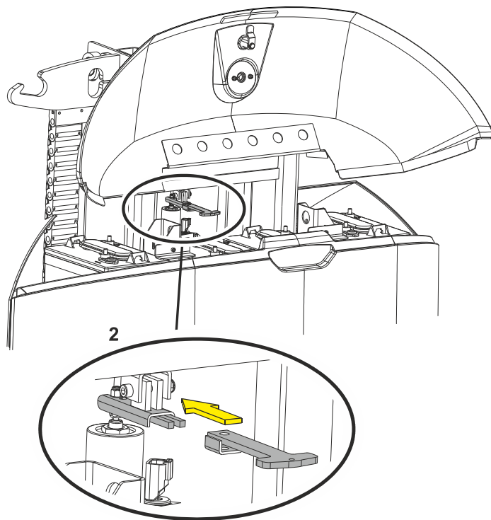
Figura 3-6. Válvula de descenso manual del mástil
