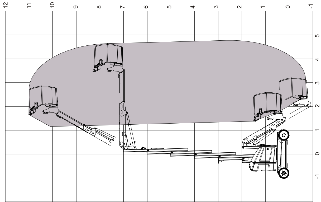
Figura 5-1. Diagrama de alcance 12E / 32E
