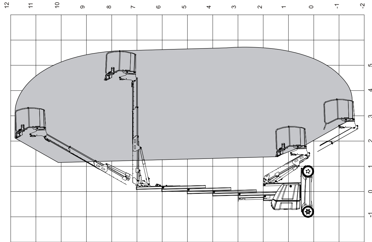
Figura 5-2. Diagrama de alcance 12E Plus
