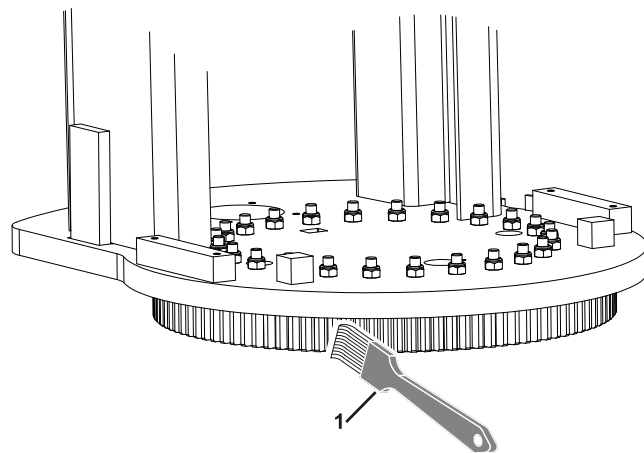
Figura 5-15. Lubricación de dos Dientes del Cojinete de Giro
