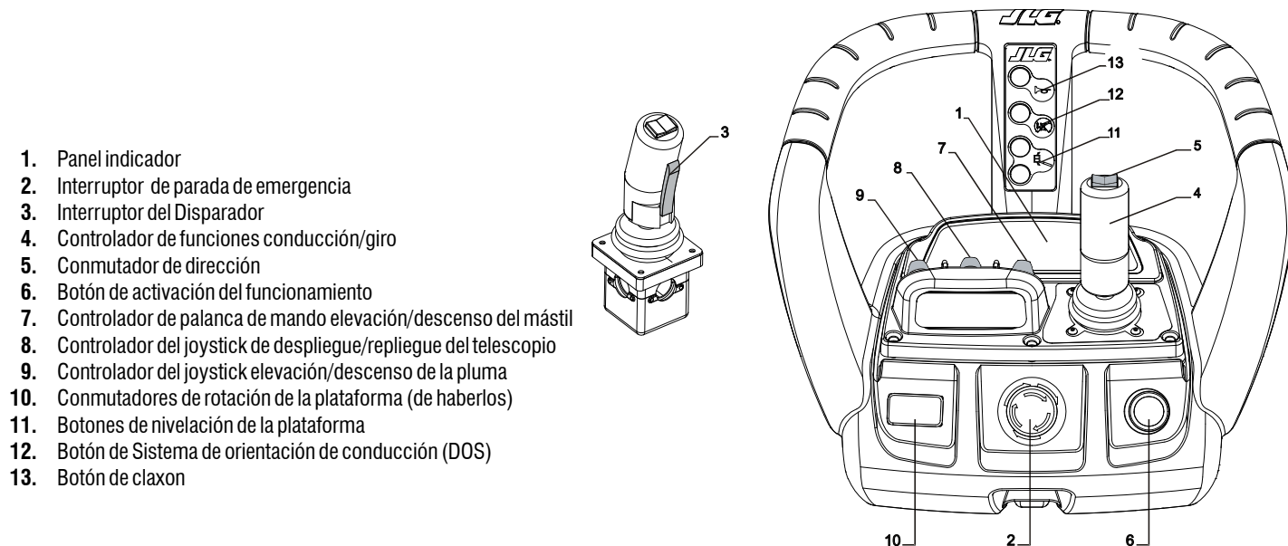
Figura 3-9. Estación de control de la plataforma
