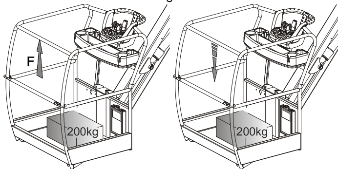
Figura 5-16. Verificación del sistema de sobrecarga
