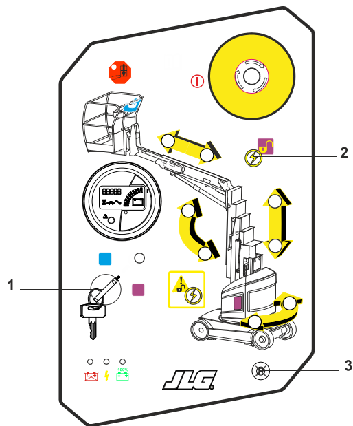
Figura 3-16. Retirada Eléctrica de los Frenos
